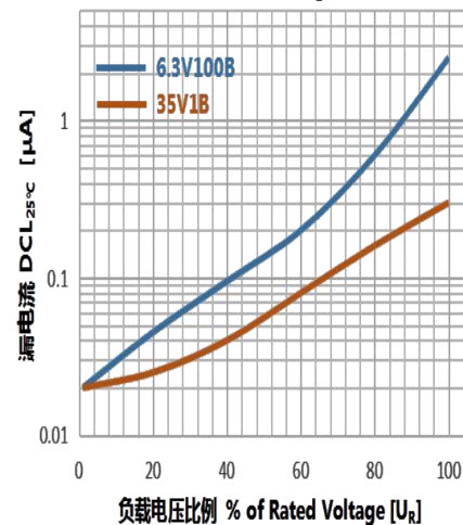
直流漏电流与负载电压的关系 DCL vs. Voltage
